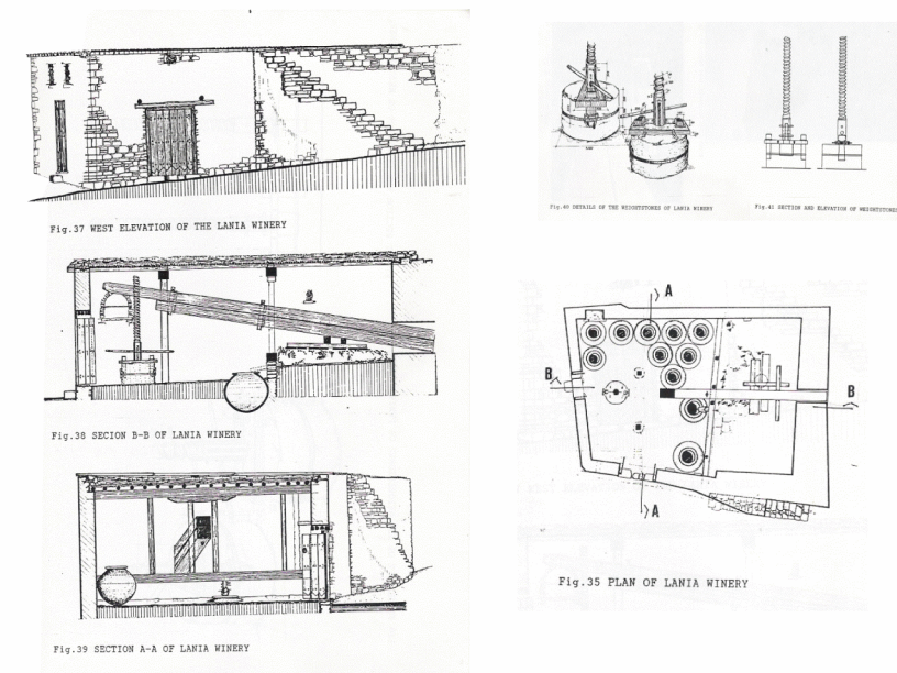
Αρχιτεκτονικά σχέδια και διαγράμματα που εξηγούν την λειτουργία του ληνού
