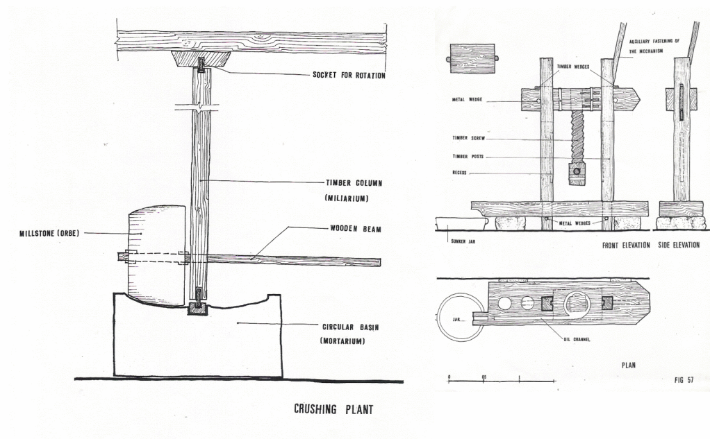
Ελαιοτριβείο ή ελιόμυλος
